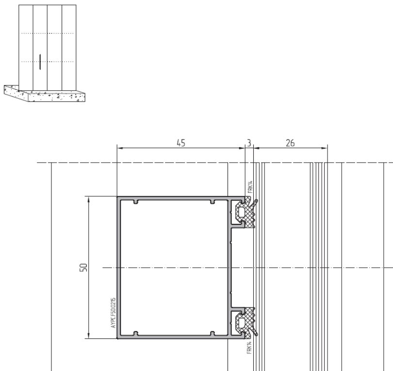
Рис. 1. Сечение фасада с использованием фальш-ригеля АУРС.F50.0215.
