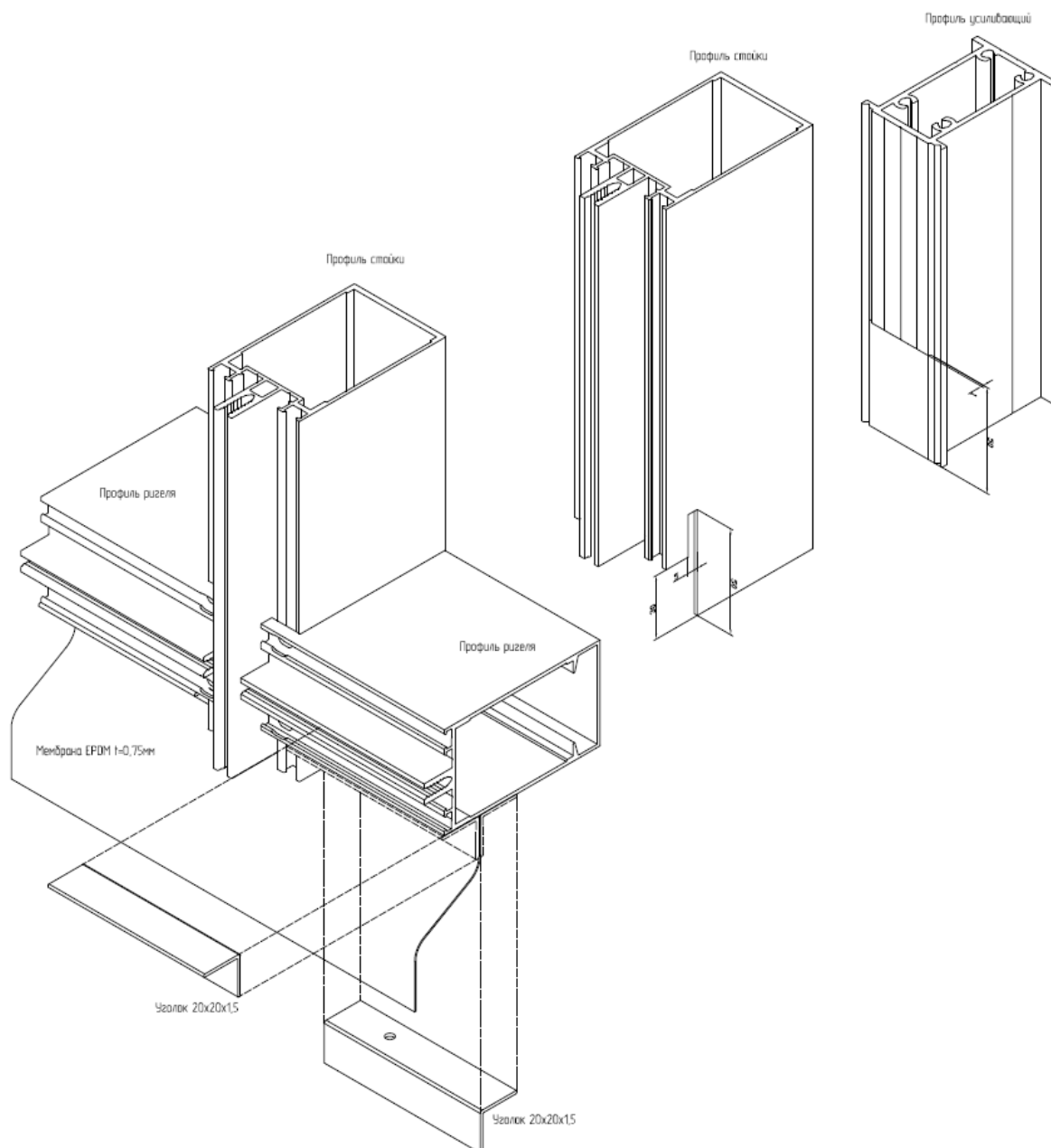
Рис. 2. Установка резинового фартука FRK150-01.
